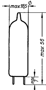
Kolbenabmessungen
